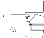
MCD' HSK-A63 F.26 PCLNR/L 065.12
