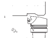
MCD' HSK-A63 F.26 PDJNR/L 070.15
