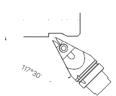
MCD' HSK-A63 F.77 SVVBN 140.16
